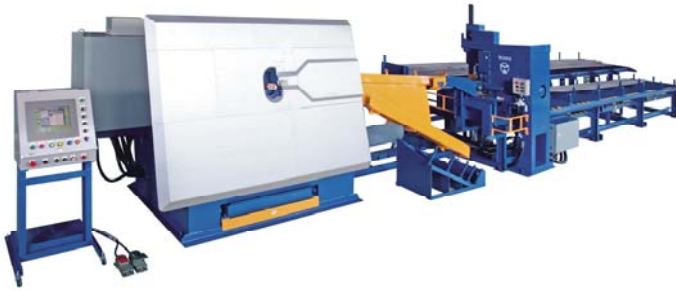
当社製品（鉄筋自動切曲げ装置）
